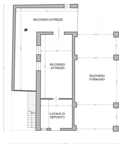
PIANTA FIENILE PIANO TERRA
