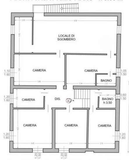
PIANTA CASA PRIMO PIANO - h 3.00 m
