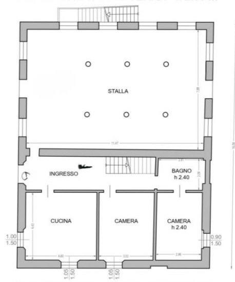
PIANTA CASA PIANO TERRA - h 2.80 m
