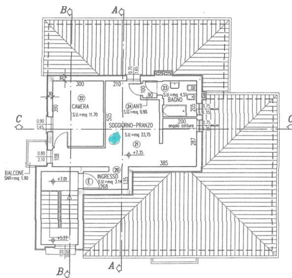
PIANTA PIANO SECONDO
